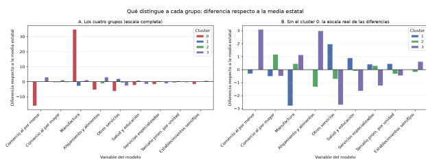
Figura 4. Perfil comparativo de variables normalizadas (Z-Score) por cluster.
