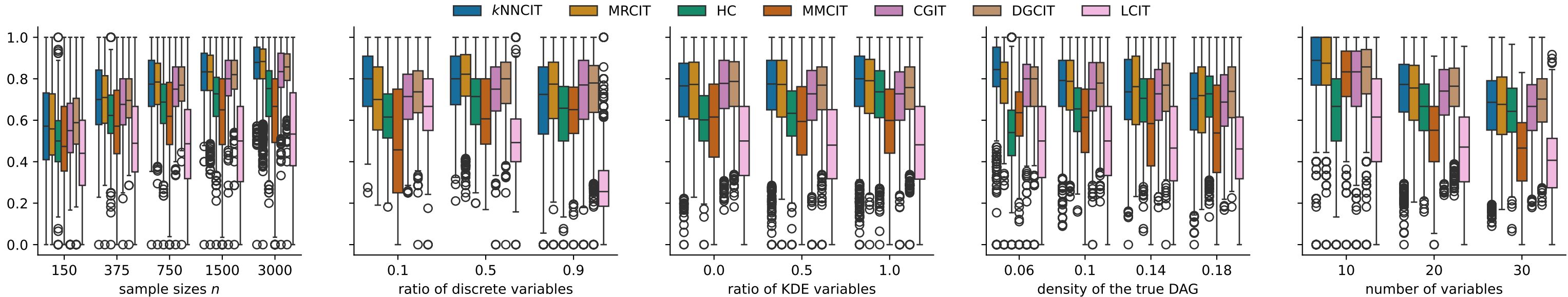
F1 score
