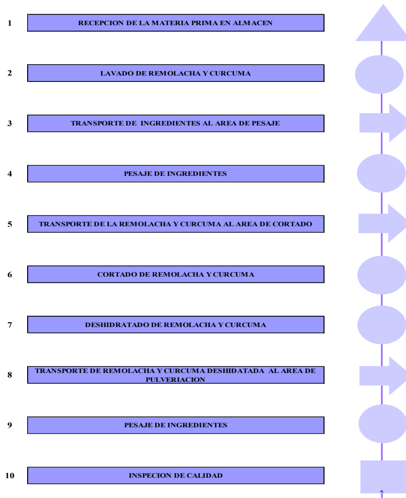
Figura 13: Flujo de proceso
