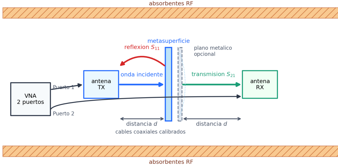
Figura 1: Montaje experimental propuesto. El diagrama separa la onda incidente, la transmisión S_{21} y la reflexión S_{11} para evitar cruces visuales. El plano metálico posterior es opcional.
