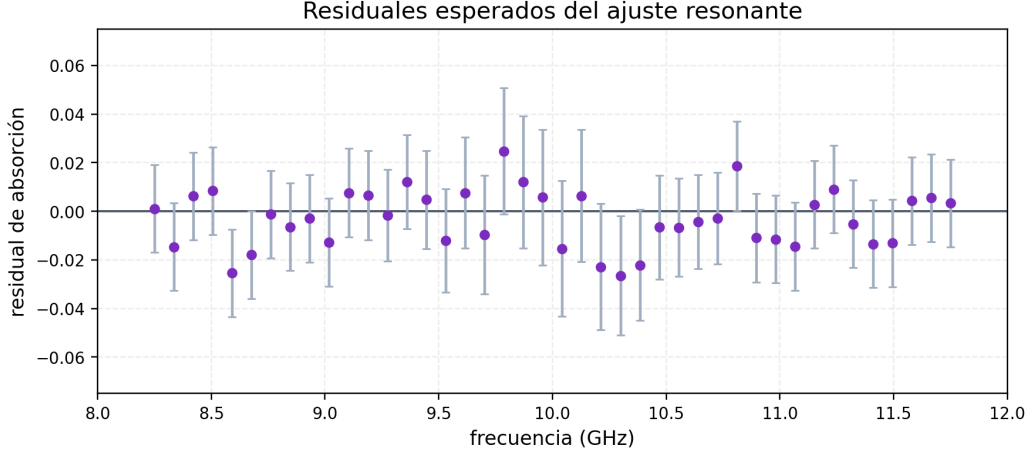
Figura 5: Residuales esperados entre datos sintéticos y ajuste resonante.
