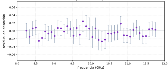
Residuales esperados del ajuste resonante
