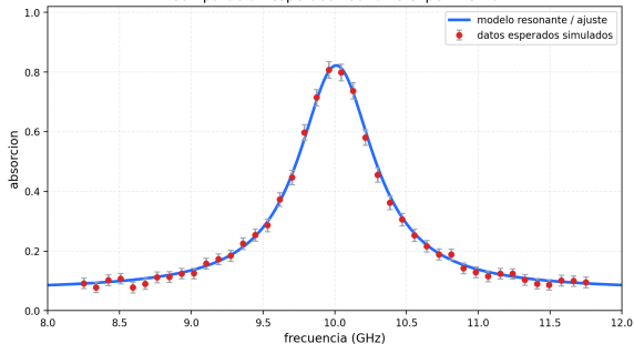
Comparacion esperada teoria vs experimento
