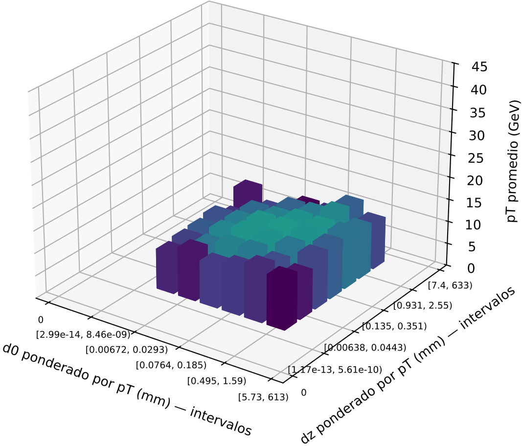
FP — N=3,221
