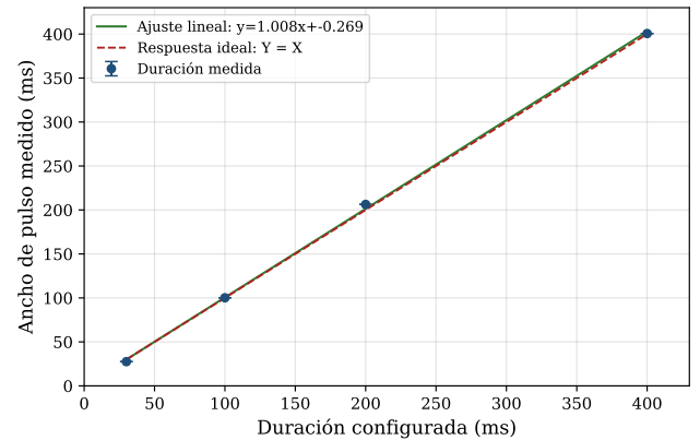
Figura 3: Relación entre el ancho de pulso programado en el LED y la duración capturada por el muestreo del ADC. La recta de tendencia uno a uno avala la cadena de medición como un reloj fiduciario confiable para el estudio asíncrono.
