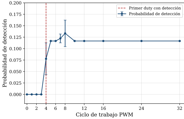
Figura 4: Evolución de la probabilidad de captura en la cámara web frente al duty cycle (baja emisión). El tope probabilístico ilustra el límite impuesto por el submuestreo, evidenciando la pérdida de la gran mayoría de los eventos.
