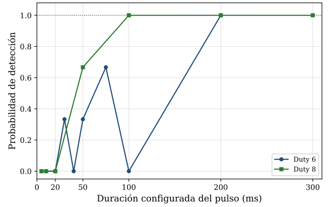
Figura 5: Mapeo probabilístico en función de la duración de emisión. La caída a cero para pulsos menores a 20 ms demuestra la incapacidad de un sensor de video estándar para caracterizar directamente eventos rápidos individuales.
