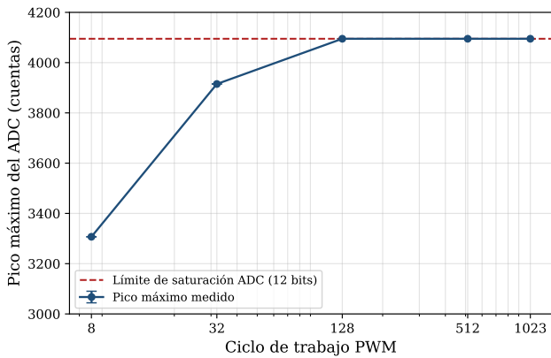
Figura 1: Respuesta de amplitud máxima en el canal OP598-ADC frente al incremento del ciclo de trabajo del LED para estímulos de 200 ms. Se evidencia la inmediata saturación del canal analógico, limitando su linealidad exclusivamente a los regímenes más bajos de intensidad.
