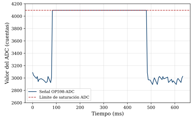
Figura 2: Registro temporal crudo de un pulso representativo detectado por el fototransistor. El rápido cruce desde el nivel basal de oscuridad hacia el techo digital reafirma la viabilidad de utilizar esta señal para fijar marcas temporales precisas.
