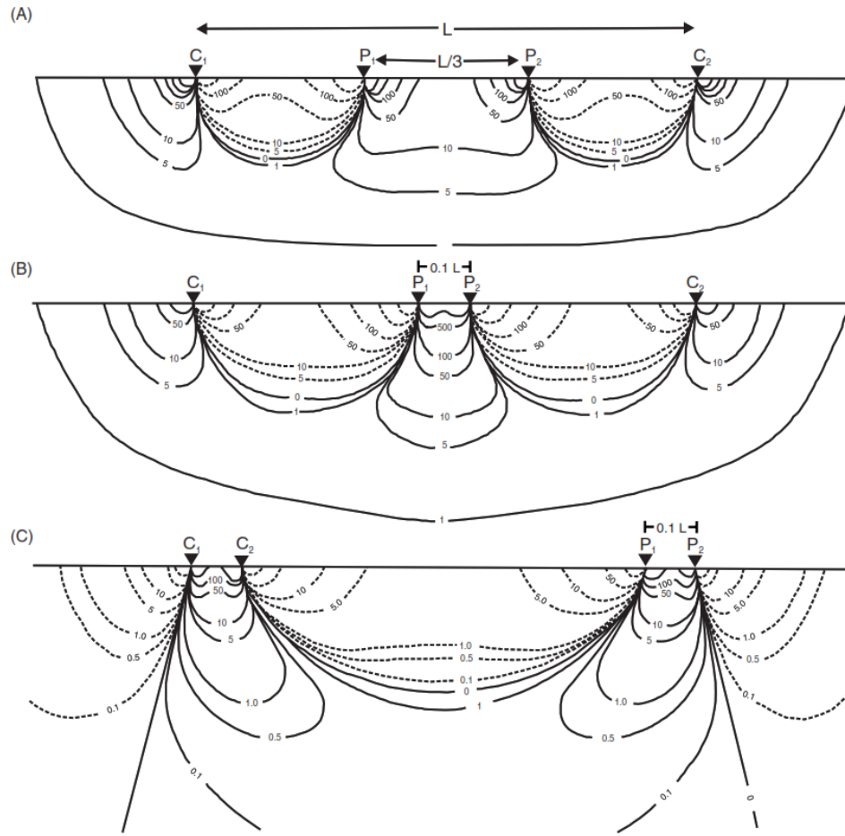
FIGURA 5.3: Esquema de la contribución de la respuesta de resistividad eléctrica, modificado de ?.
