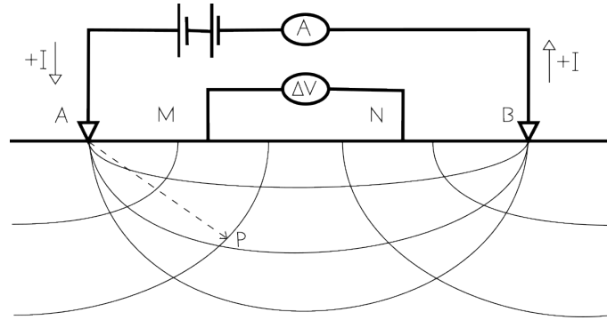
FIGURA 5.2: Configuración general de arreglo de electrodos, modificado de ?.
