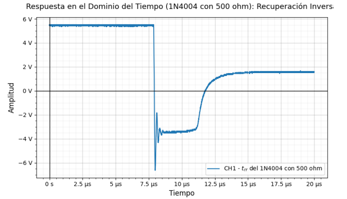
Figura 14: Muestra del t_{rr} del diodo 1N4004 con R = 500\Omega
