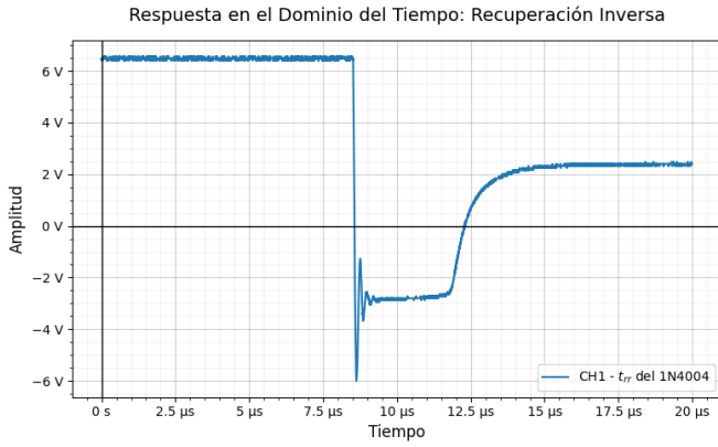
Figura 12: Muestra del t_{rr} del diodo 1N4004 a 10 kHz
