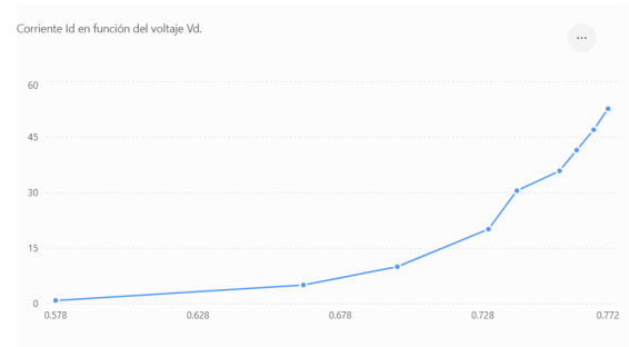
Figura 10: Gráfica I_D vs V_D para el diodo 1N4004
