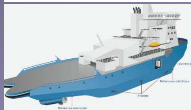
Sistema ICCP Cathelco® para rompehielos
