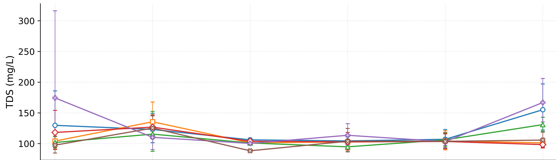
Serie temporal de SDT
