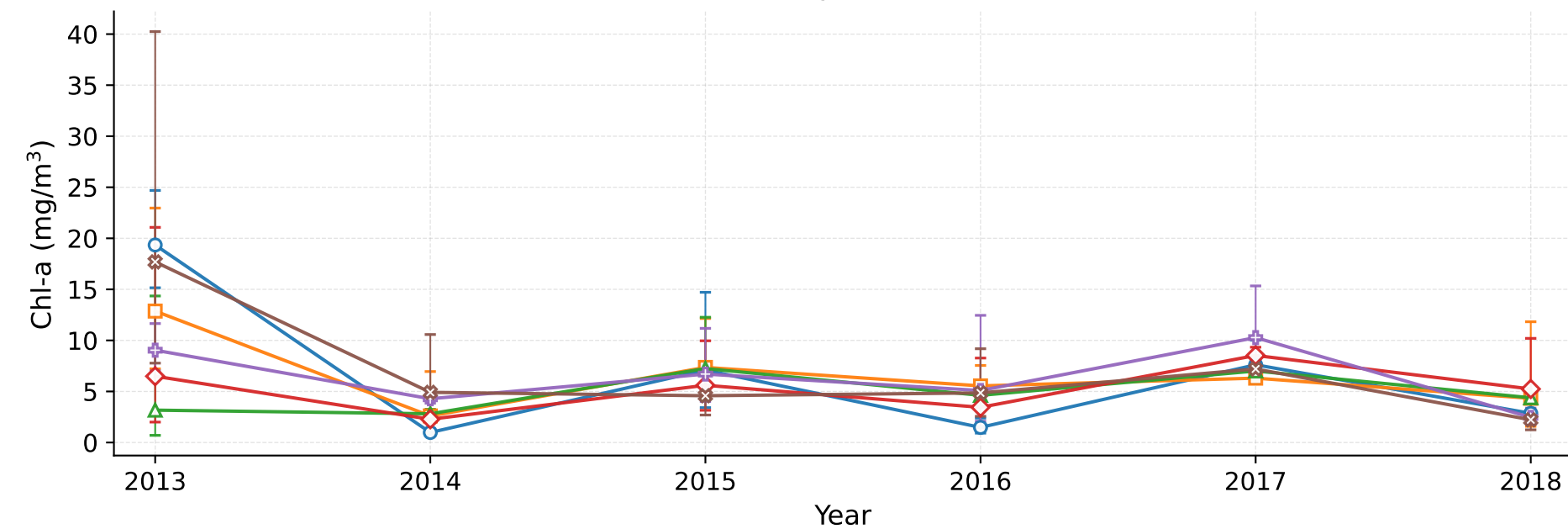
Serie temporal de Cl-a
