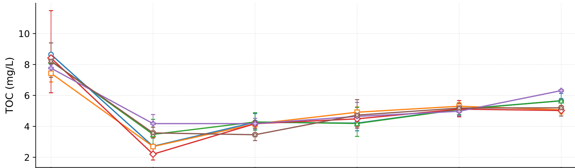
Serie temporal de COT
