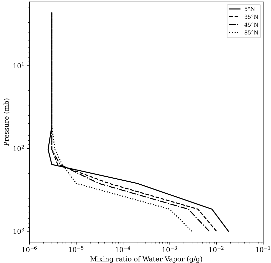
Fig 5a: H_2O Latitudinal Variation
