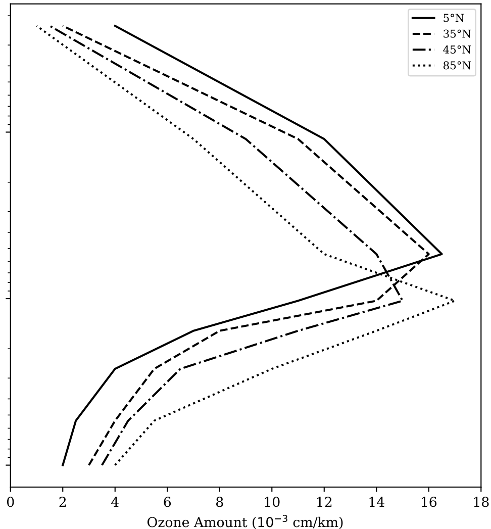
Fig 5b: O_3 Latitudinal Variation
