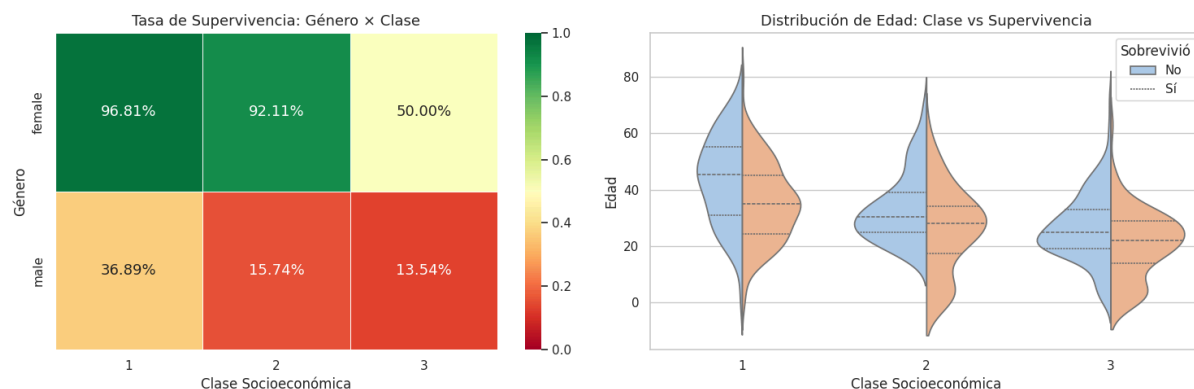
Figura 5. Heatmap de supervivencia por género y clase (izquierda) y violin plot de edad por clase y supervivencia (derecha).
