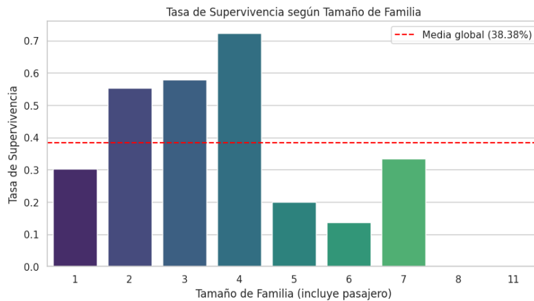
Figura 8. Tasa de supervivencia según el tamaño del grupo familiar. La línea roja indica la media global (38.4%).
