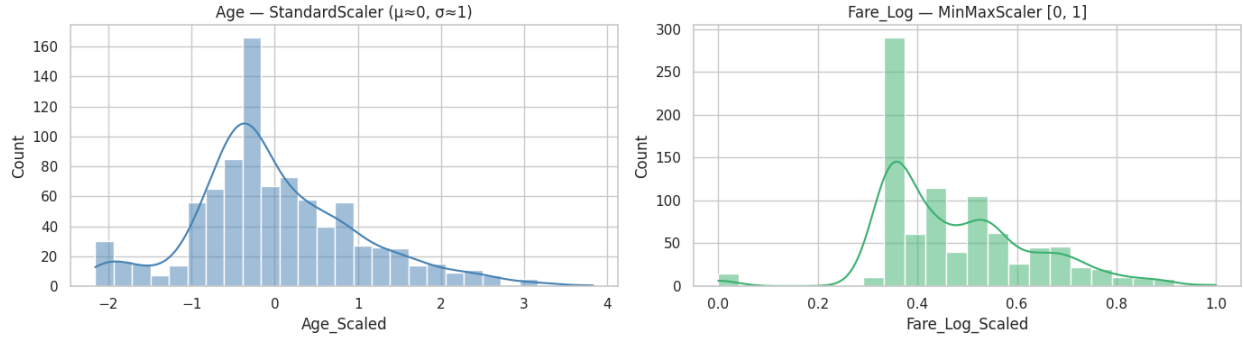
Figura 7. Verificación visual de las distribuciones tras el escalamiento de Age (izquierda) y Fare_Log (derecha).
