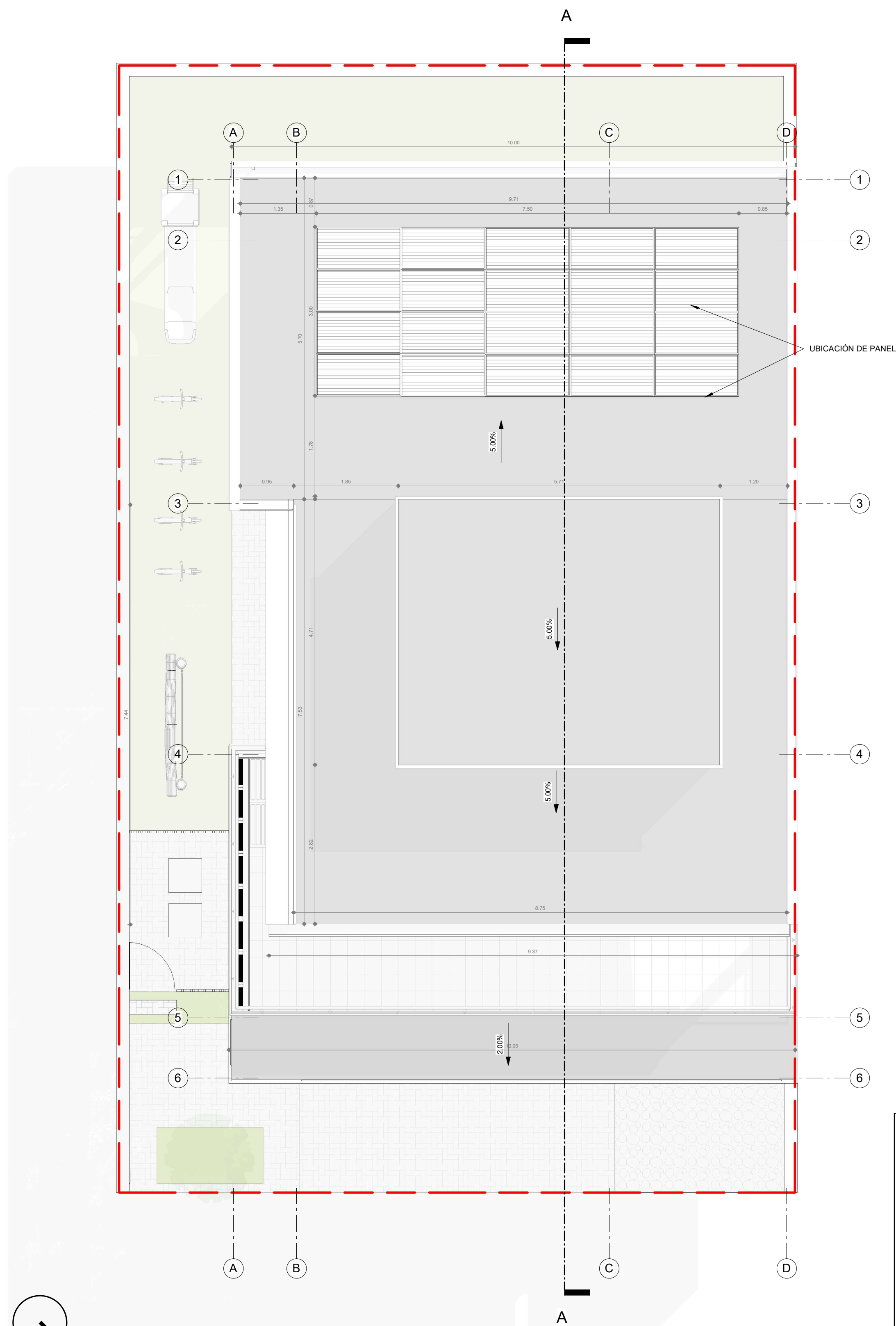
AQ05 Planta de Cubiertas ESC: 1 : 50
