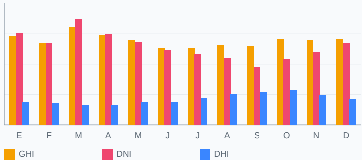
b) Radiación solar mensual
