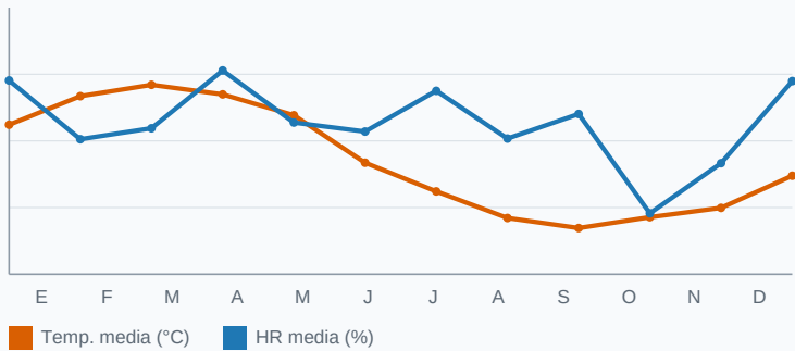
a) Temperatura y humedad relativa mensual
