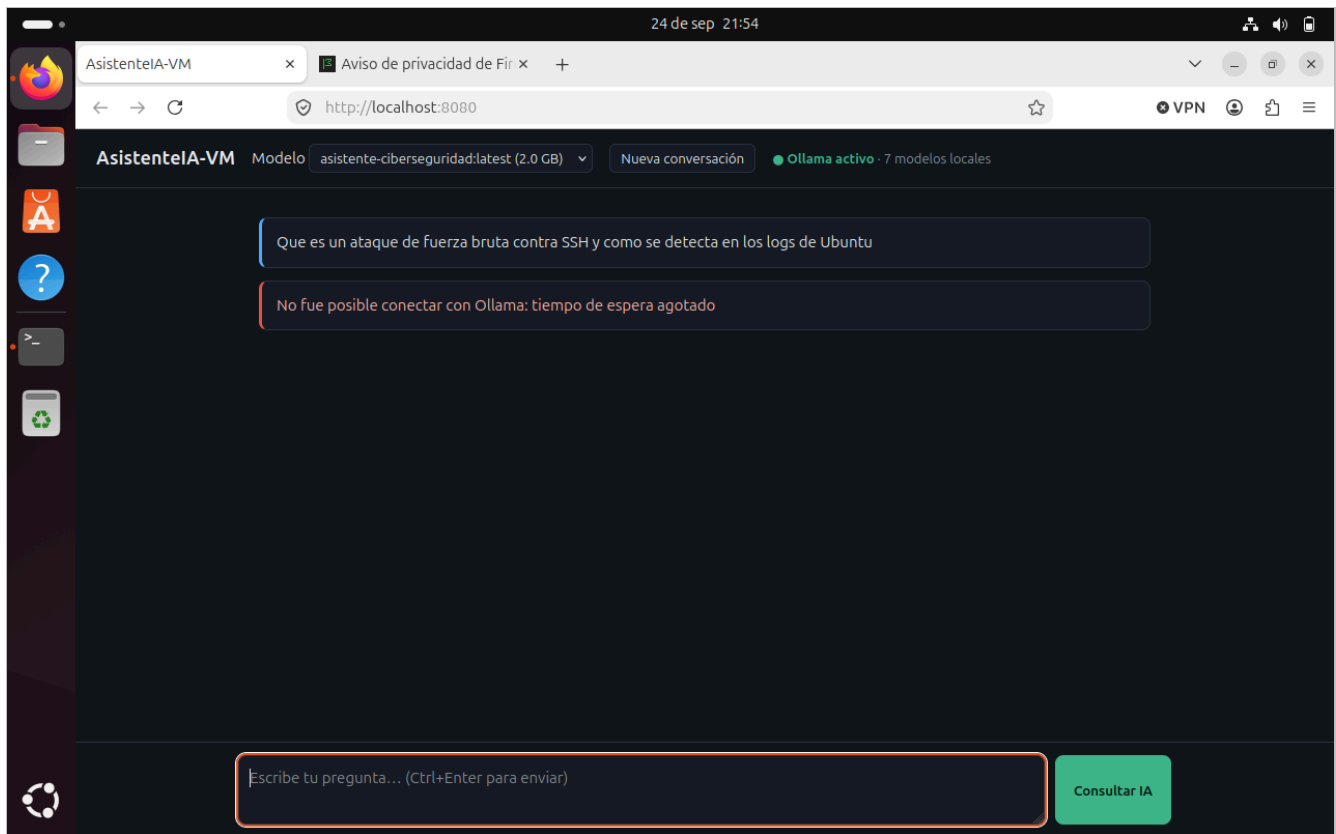
Captura 9. Primera versión (sin streaming, límite total de 5 min). Con Firefox abierto la VM generaba a solo 2,3 tok/s y la respuesta pasaba de 560 tokens, así que se agotó el tiempo. El manejo de errores funcionó, pero el usuario no veía nada durante 5 minutos. Por eso se pasó a streaming.
