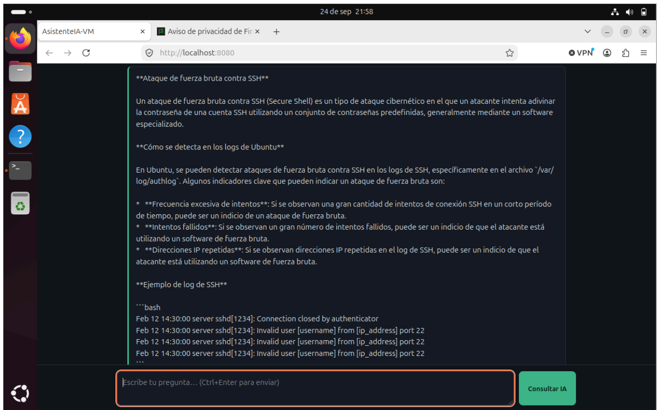
Captura 8. Primera respuesta del asistente sobre ataques de fuerza bruta contra SSH. Ya aquí aparece la ruta equivocada /var/log/authlog , que se valida más abajo.
