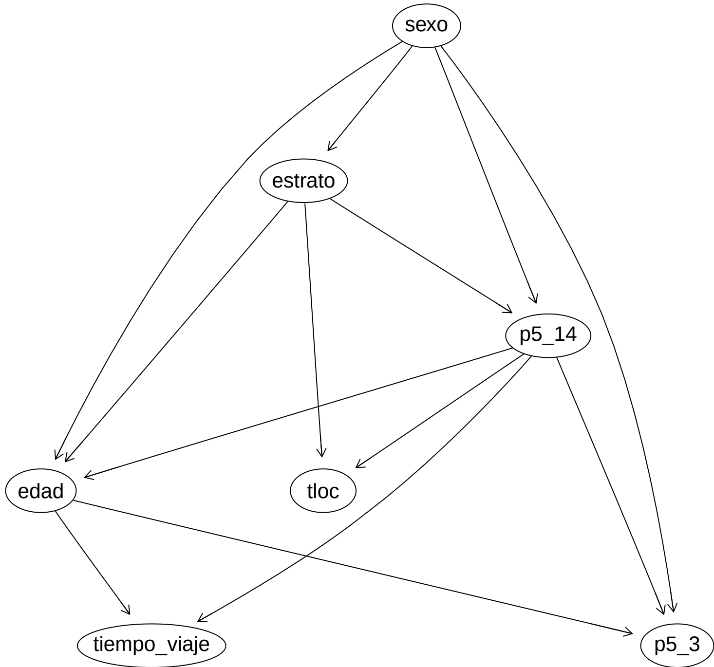
Mejor DAG (Hill Climbing)
