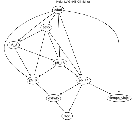
Figure 4: Mejor DAG obtenido por Hill Climbing
