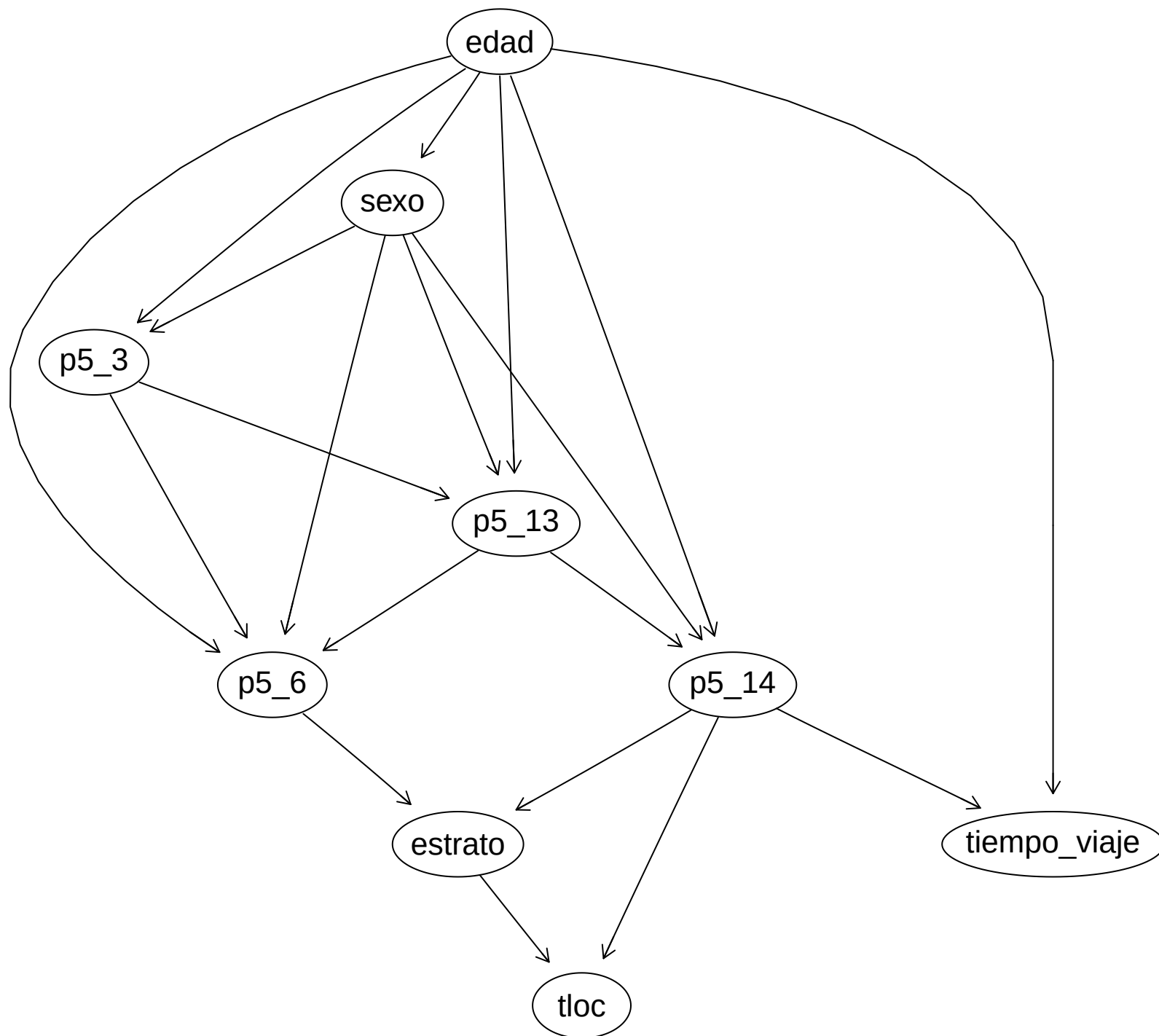
Mejor DAG (Hill Climbing)
