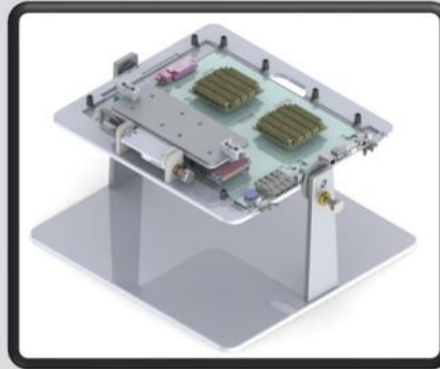
Fixtura de giro para soldado manual e inspección
