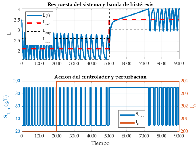
Figura 5c. Control On-Off para S_{1,in} con I_0 .
