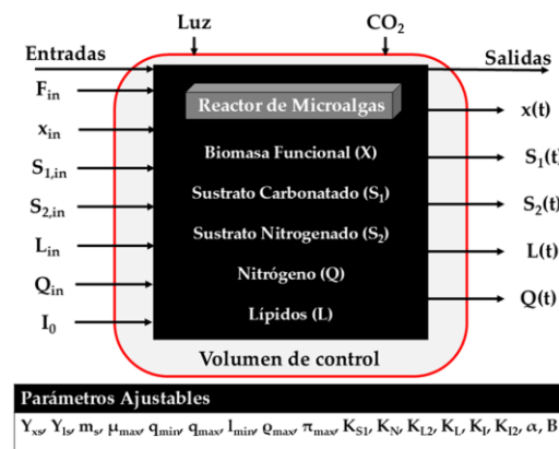
Figura 1. Diagrama de caja negra
