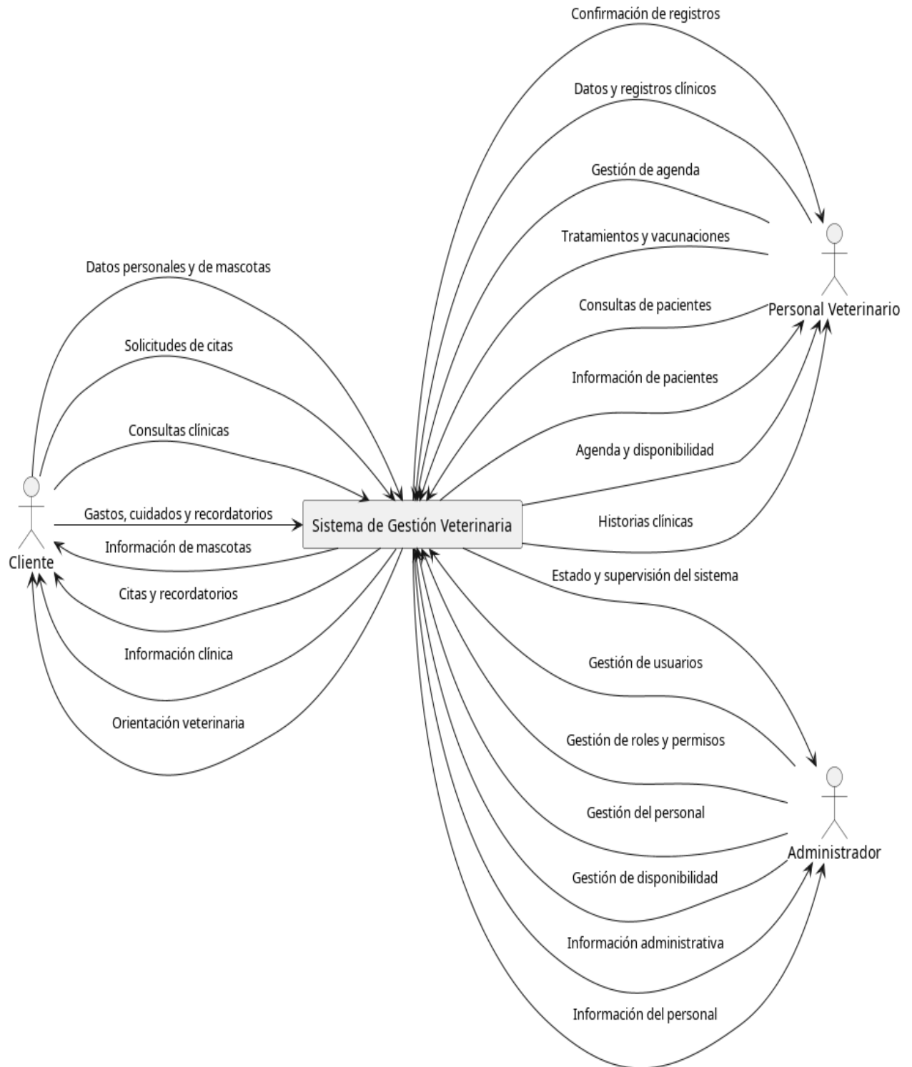
Diagrama de Contexto - Sistema de Gestión Veterinaria
