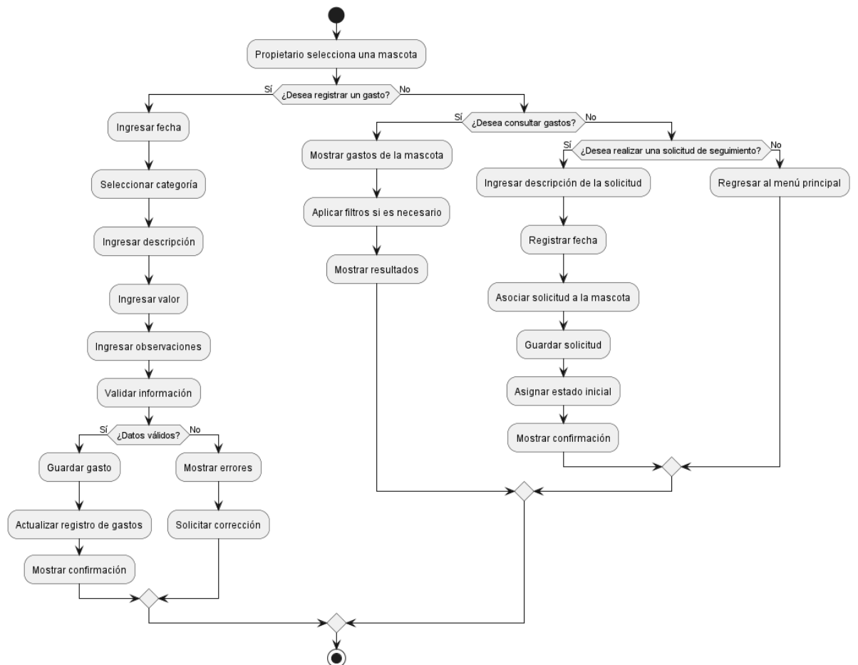
Diagrama de flujo 5 - Gastos y solicitudes de seguimiento
