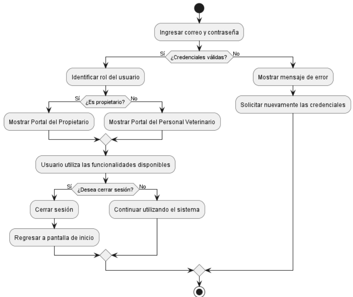
Diagrama de flujo 1 - Autenticación y acceso
