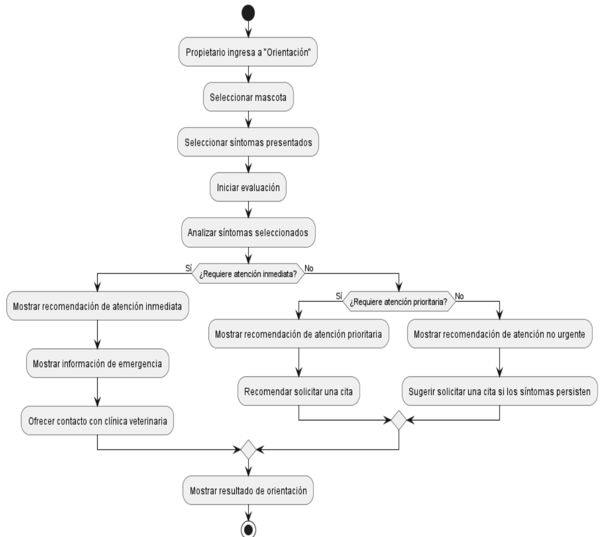
Diagrama de flujo 6 - Orientación ante síntomas y emergencias
