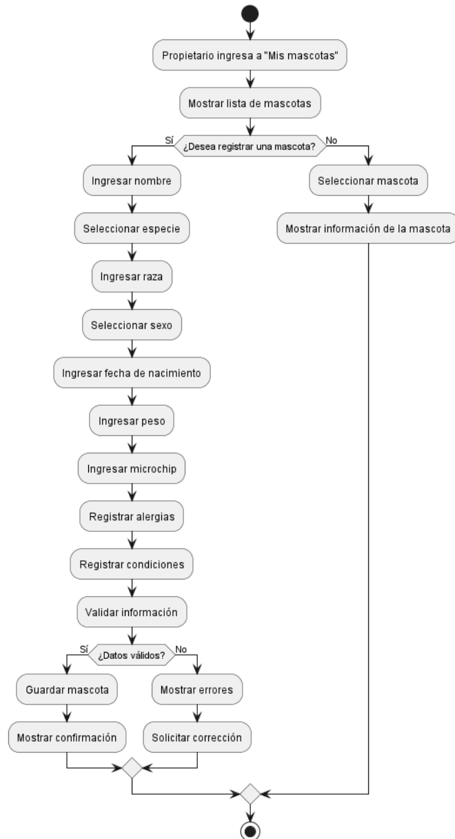
Diagrama de flujo 2 - Gestión de mascotas
