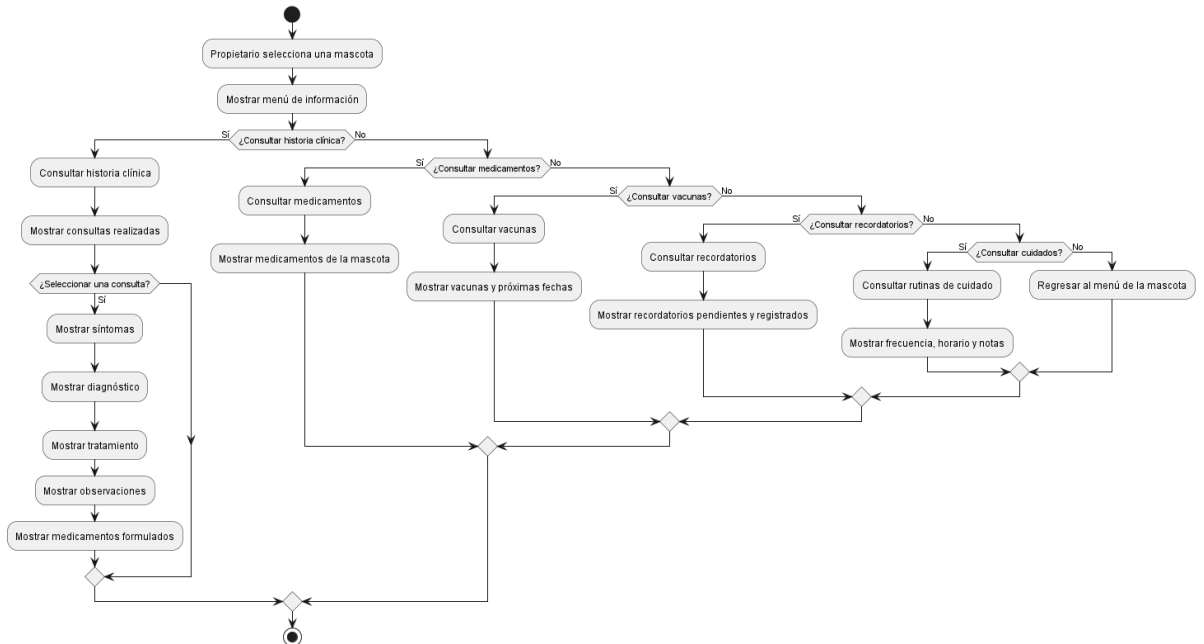
Diagrama de flujo 4 - Consulta de información clínica y cuidados
