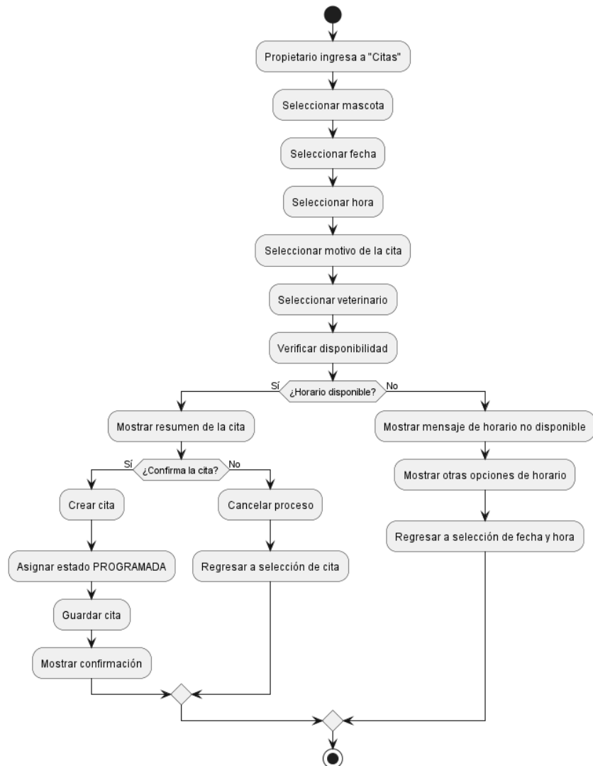
Diagrama de flujo 3 - Agendamiento de citas
