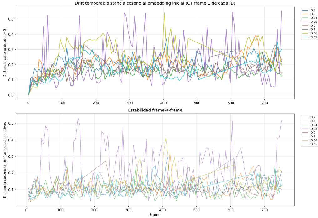
Figura 16: Evolución temporal de la distancia respecto al embedding inicial. En general, las curvas se mantienen bajas, lo que indica una estabilidad temporal razonable del descriptor visual para una misma trayectoria.
