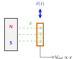
Figura 6.9: Transductor electrodinámico. La tensión de salida es una réplica exacta de la velocidad instantánea del objeto, muy común en sismometría y monitorización de turbinas.
