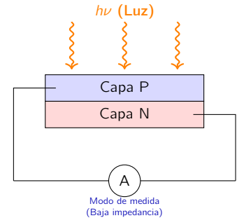
Figura 6.8: Operación de un sensor fotovoltaico. La energía de los fotones genera portadores de carga que dan lugar a la corriente de fotodiodo I_{ph} .
