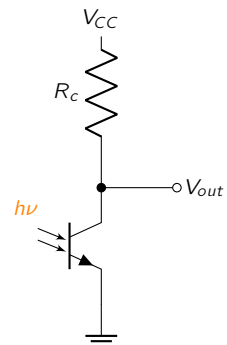
Figura 7.6: Fototransistor en configuración de emisor común. La ganancia \beta proporciona una señal de salida robusta a cambio de una menor velocidad de conmutación.
