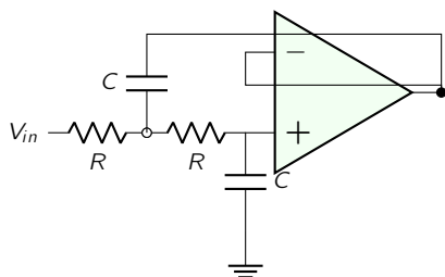
Figura 5.3: Filtro paso bajo Sallen-Key de segundo orden. Presenta una caída de 40 dB/decada tras la frecuencia de corte.
