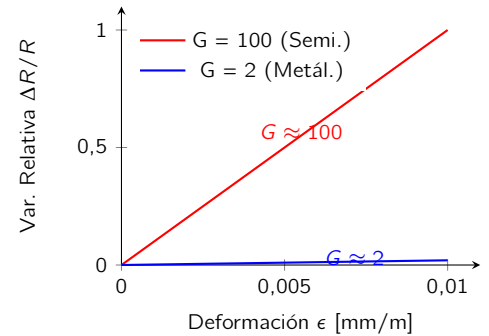
Figura 3.3: Comparativa de sensibilidad entre galgas. Nótese que para una deformación de 0,01 mm/m, la galga metálica apenas varía un 2 %, mientras que la de semiconductor llega al 100 % de variación ( \Delta R = R ).
