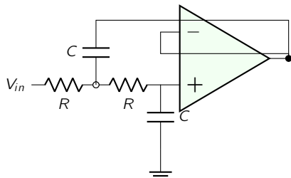
Figura 5.4: Filtro activo paso bajo Sallen-Key de segundo orden equivalente al filtro RLC pasivo. Presenta una caída de 40 dB/decada tras la frecuencia de corte.
