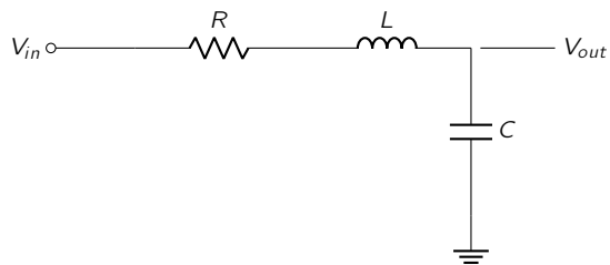
Figura 5.3: Filtro pasivo RLC paso bajo convencional.
