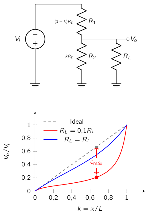
Figura 3.2: Efecto de carga. El circuito (arriba) muestra la R_L en paralelo con el brazo inferior. La gráfica (abajo) ilustra cómo la salida se aplasta respecto a la ideal, perdiendo linealidad. El eje y representa la relación V_o/V_i y el eje x la posición del cursor.
