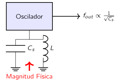
Figura 4.21: Acondicionamiento mediante conversión a frecuencia. El sensor forma parte de la red de realimentación de un oscilador.
