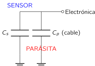
Figura 4.6: Efecto de la capacidad parásita del cable. C_p aparece en paralelo con el sensor, sumándose a la medida y reduciendo drásticamente la variación relativa \Delta C/C_{total} .
