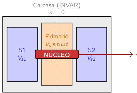
Figura 4.15: Sección transversal del LVDT. El primario está alimentado con una señal alterna. Las dos secundarias están conectadas en oposición de serie. La varilla de accionamiento controla la posición del núcleo ferromagnético. El núcleo ferromagnético se encuentra en la sección transversal.
