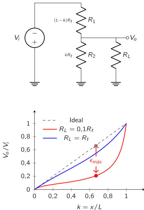
Figura 3.2: Efecto de carga. El circuito (arriba) muestra la R_L en paralelo con el brazo inferior. La gráfica (abajo) ilustra cómo la salida se aplata respecto a la ideal, perdiendo linealidad. El eje y representa la relación V_o/V_i y el eje x la posición del cursor.
