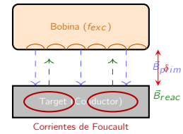
Figura 4.17: Principio de los sensores de corrientes de Foucault. Las corrientes inducidas en el target crean un campo de reacción que modifica la impedancia de la bobina como función de \delta .
