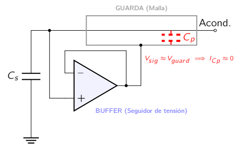
Figura 4.8: Esquema de guarda activa. El buffer de ganancia unidad asegura que la malla del cable esté al mismo potencial que el hilo de señal ( V_{sig} \approx V_{guard} ), eliminando la corriente a través de C_p . Al no haber diferencia de tensión entre los terminales de C_p , esta capacidad no se carga ni descarga, eliminando su efecto en la medida del sensor.
