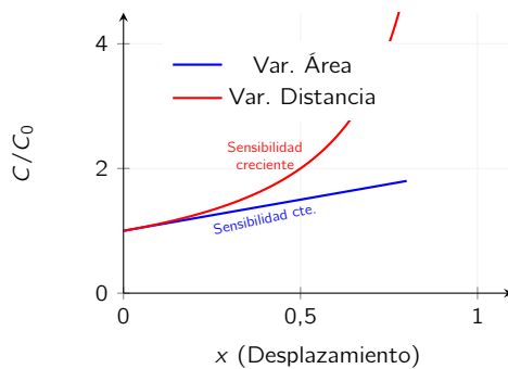
Figura 4.4: Comparativa de respuesta. El sensor de distancia es ideal para desplazamientos ínfimos (nanómetros), mientras que el de área es preferible para rangos mayores.
