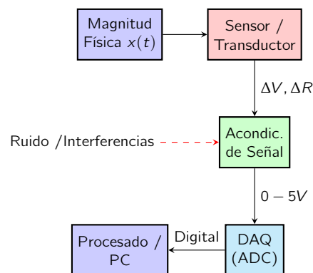
Figura 1.1: Cadena de Instrumentación: Desde la magnitud física hasta la información útil. La magnitud física se transforma en una señal eléctrica mediante un sensor o transductor. La señal eléctrica se acondiciona para mejorar la calidad de la señal y se transforma en digital. La señal digital se adquiere mediante un sistema de adquisición. La información digital se procesa y se presenta.
