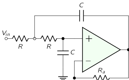
Figura 5.4: Filtro activo paso bajo Sallen-Key de segundo orden equivalente al filtro RLC pasivo. Presenta una caída de 40 dB/década tras la frecuencia de corte.
