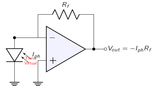
Figura 7.5: Acondicionamiento típico de un fotodiodo ( Transimpedance Amplifier , TIA). El operacional mantiene el diodo en modo fotovoltaico (tensión nula) para maximizar la linealidad.
