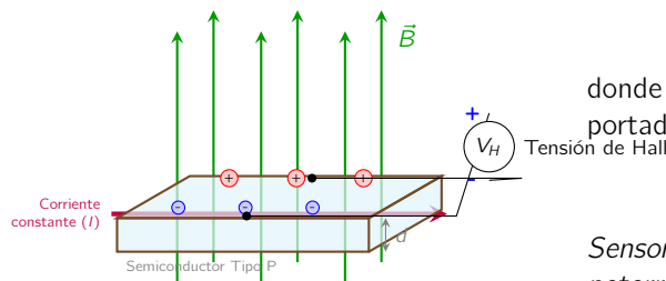
Figura 4.19: Principio del efecto Hall. El campo magnético \vec{B} atraviesa verticalmente el material. La fuerza de Lorentz desvía los portadores mayoritarios (huecos en tipo P) hacia la cara posterior, estableciendo una diferencia de potencial transversal V_H .
