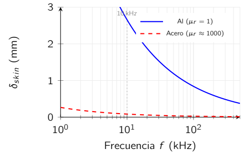
Figura 4.18: Profundidad de penetración \delta_{skin} frente a frecuencia de excitación para aluminio y acero. El acero, al ser ferromagnético ( \mu_r \gg 1 ), confina las corrientes en una capa mucho más delgada.
