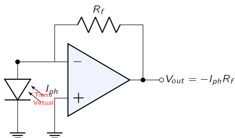
Figura 7.3: Acondicionamiento típico de un fotodiodo (TIA). El operacional mantiene el diodo en modo fotovoltaje (tensión nula) para maximizar la linealidad.
