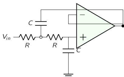
Figura 5.2: Filtro paso bajo Sallen-Key de segundo orden. Presenta una caída de 40 dB/decada tras la frecuencia de corte.
