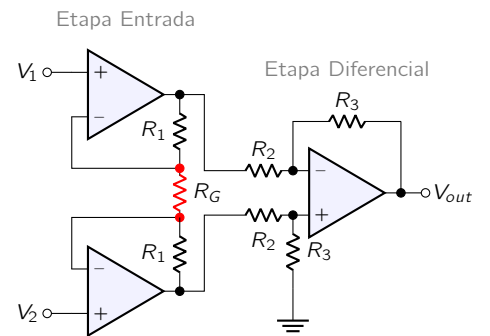
Figura 5.1: Amplificador de instrumentación de tres operacionales. La primera etapa proporciona alta impedancia y ganancia diferencial, mientras que la segunda etapa (restadora) elimina el modo común.
