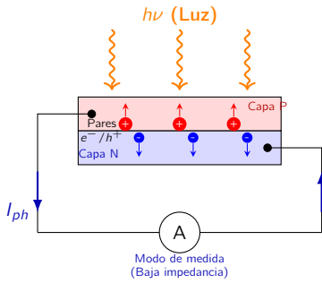
Figura 6.9: Operación de un sensor fotovoltaico. La energía de los fotones genera portadores de carga que dan lugar a la corriente de fotodiiodo I_{ph} .
