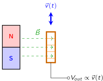
Figura 6.10: Transductor electrodinámico. La tensión de salida es una réplica exacta de la velocidad instantánea del objeto, muy común en sismometría y monitorización de turbinas.
