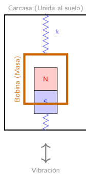
Figura 6.11: Estructura interna de un geófono. La inercia de la masa suspendida permite medir la velocidad de vibración de la carcasa.
