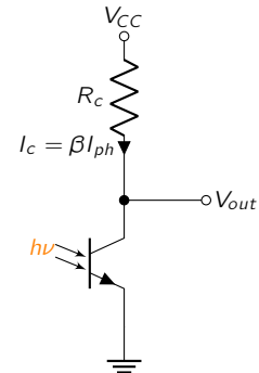
Figura 7.6: Fototransistor en configuración de emisor común. La ganancia \beta proporciona una señal de salida robusta a cambio de una menor velocidad de conmutación.
