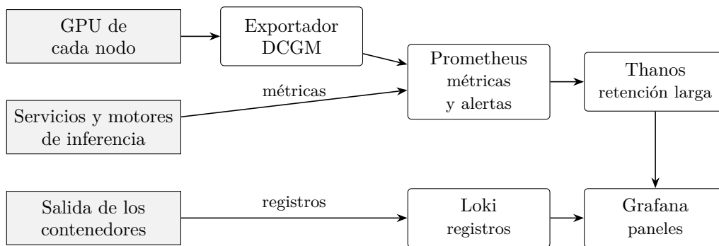
Figura 4.3: Flujo de la telemetría en el clúster. Prometheus recolecta las métricas que exponen los servicios y, a través del exportador DCGM, las de las GPU; Thanos conserva esas series a largo plazo; Loki agrega los registros de los contenedores, y Grafana presenta esas fuentes en paneles. Elaboración propia.
