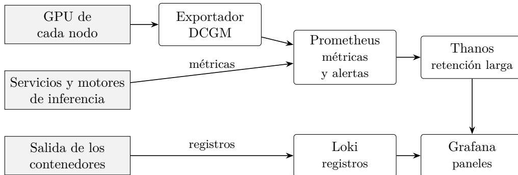
Figura 4.3: Flujo de la telemetría en el clúster. Prometheus recolecta las métricas que exponen los servicios y, a través del exportador DCGM, las de las GPU; Thanos conserva esas series a largo plazo; Loki agrega los registros de los contenedores, y Grafana presenta esas fuentes en paneles. Elaboración propia.
