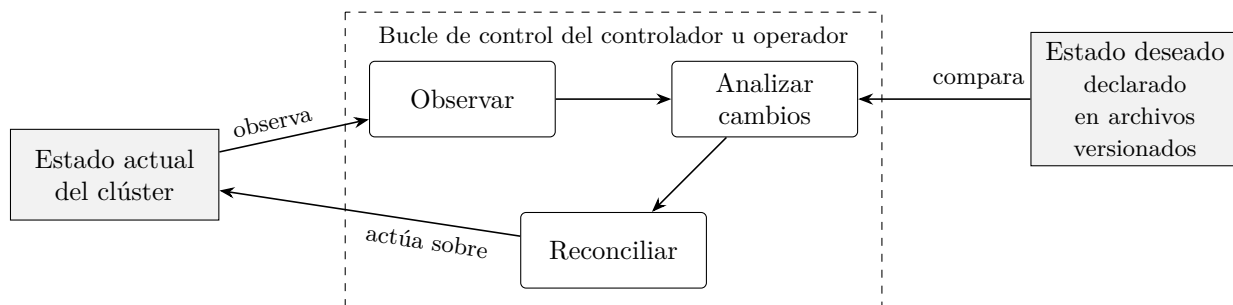
Figura 4.2: Bucle de reconciliación de un controlador de Kubernetes. El controlador observa el estado actual del clúster, lo compara con el estado deseado y actúa hasta hacerlos converger. Adaptado de Xu et al. (2024) (Figura 1) y de Burns et al. (2016).
