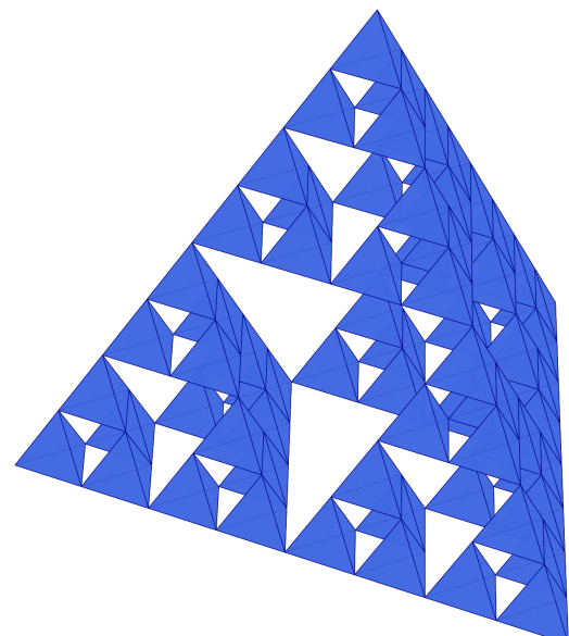
Figura 1: Construcción iterativa del Triángulo de Sierpinski Figura 2: Construcción iterativa del Tetraedro de Sierpinski
