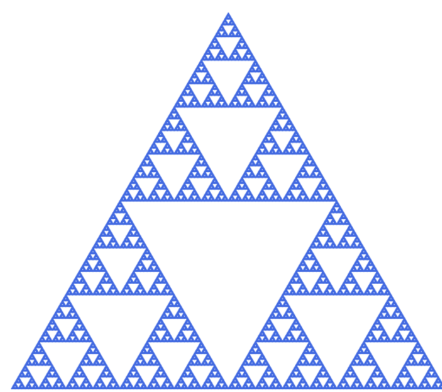
Figura 1: Construcción iterativa del Triángulo de Sierpinski Figura 2: Construcción iterativa del Tetraedro de Sierpinski
