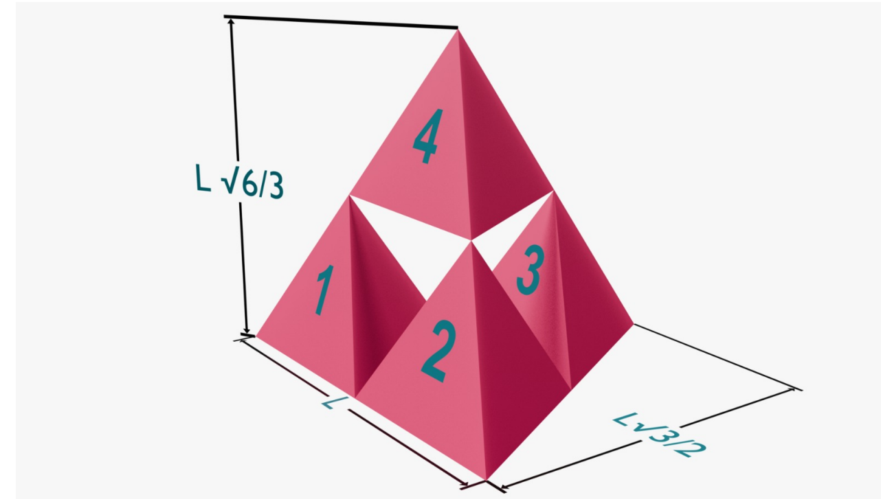
Figura 5: Orden de formación de un Tetraedro de Sierpinski
