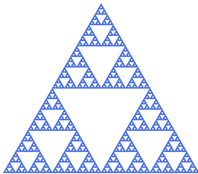
Figura 1: Construcción iterativa del Triángulo de Sierspinski
