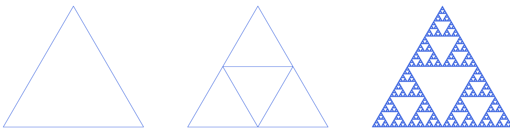
Figura 3: Triángulo de Sierpinski. Dimensión fractal: D_H \approx 1,585 .
