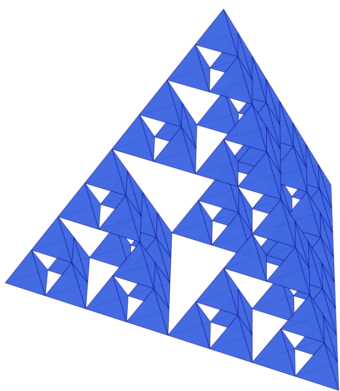
Figura 2: Construcción iterativa del Tetraedro de Sierspinski
