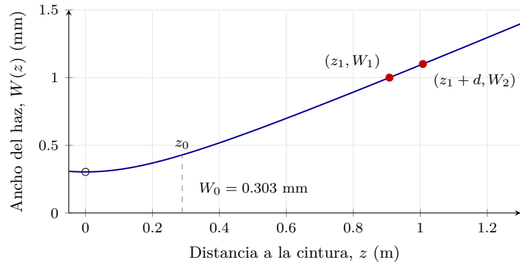
Figura 6: Ejercicio 3.1-4: ancho del haz gaussiano en función de la distancia a la cintura, con \lambda = 1 \mu\text{m} , W_0 = 0.303 mm y z_0 = 0.289 m. Se marcan el punto dado (z_1, W_1) y el punto pedido (z_1 + d, W_2) .
