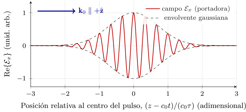
Figura 1: Instantánea del campo eléctrico del punto 1 a lo largo del eje de propagación, para un valor ilustrativo \nu_0\tau = 3 (en el óptico \nu_0\tau \gg 1 y hay muchos más ciclos bajo la envolvente). El campo oscila a lo largo de \hat{\mathbf{x}} y el pulso completo avanza en +z con velocidad c_0 .
