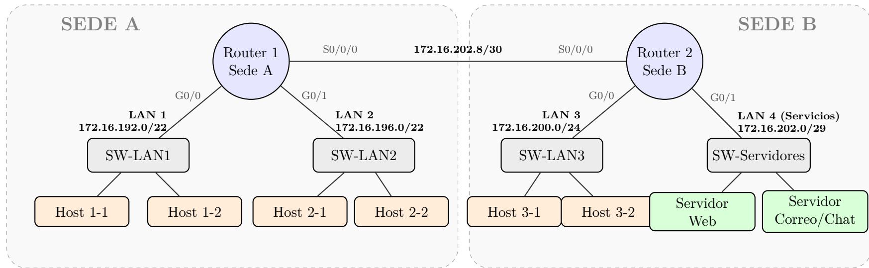
Figura 2: Topología lógica con asignación de interfaces y subredes IPv4
