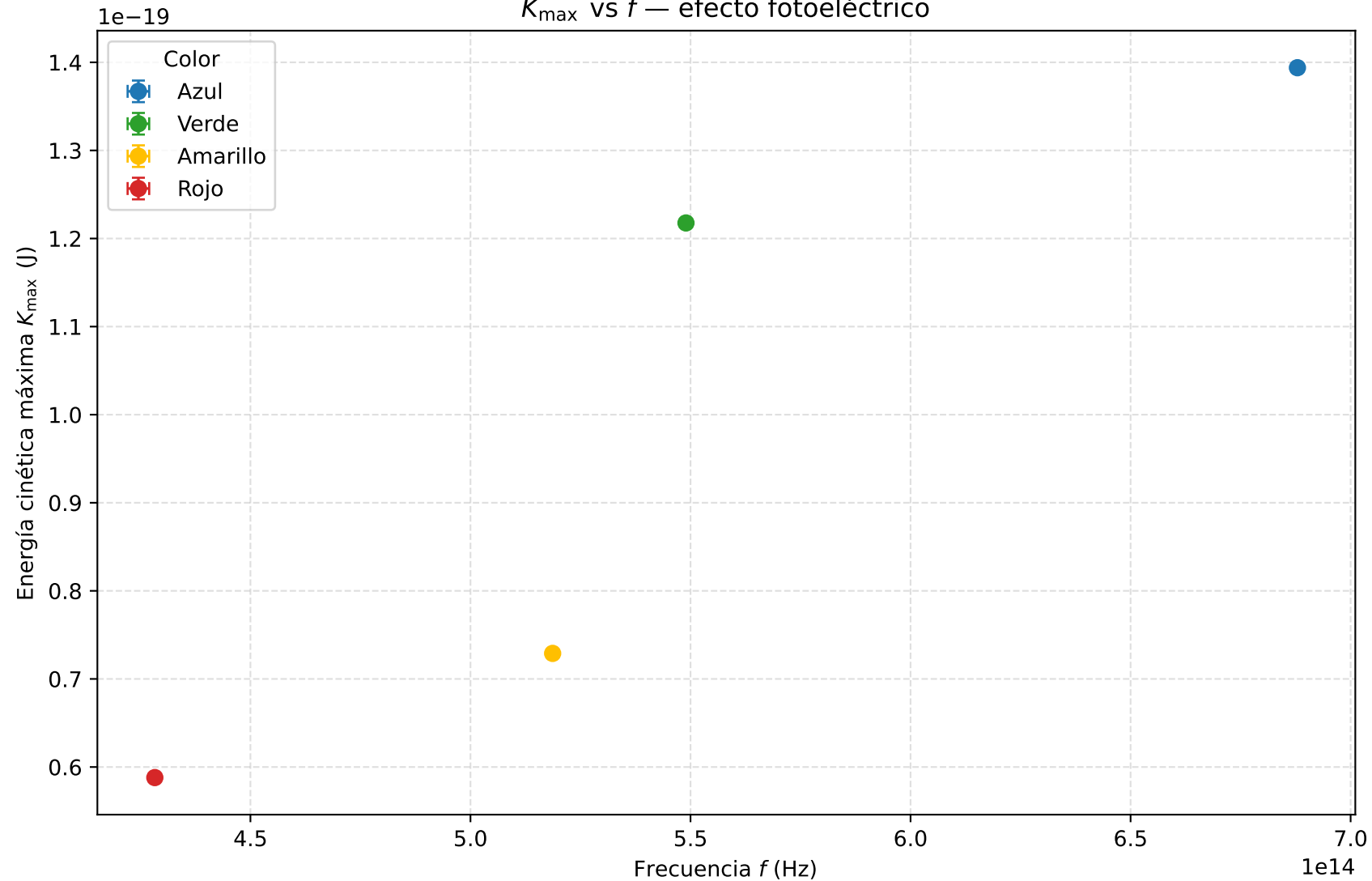
K_{\max} vs f — efecto fotoeléctrico
