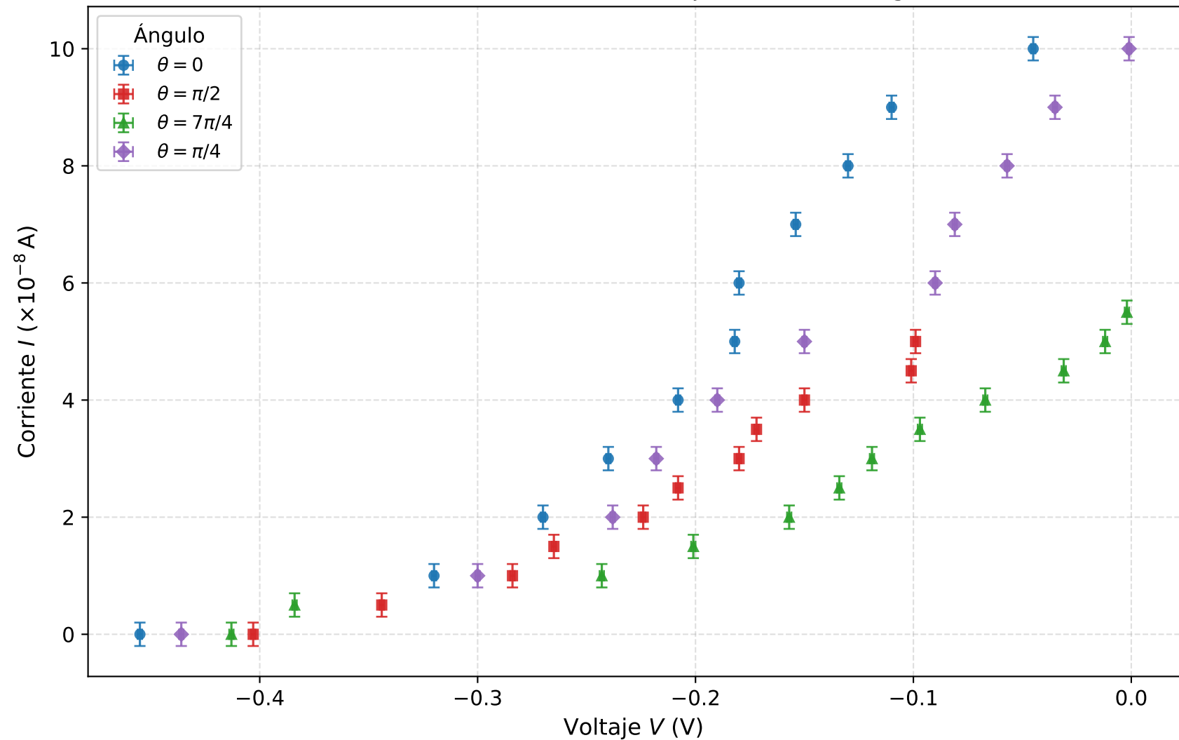
Luz amarilla: corriente vs voltaje a distintos ángulos
