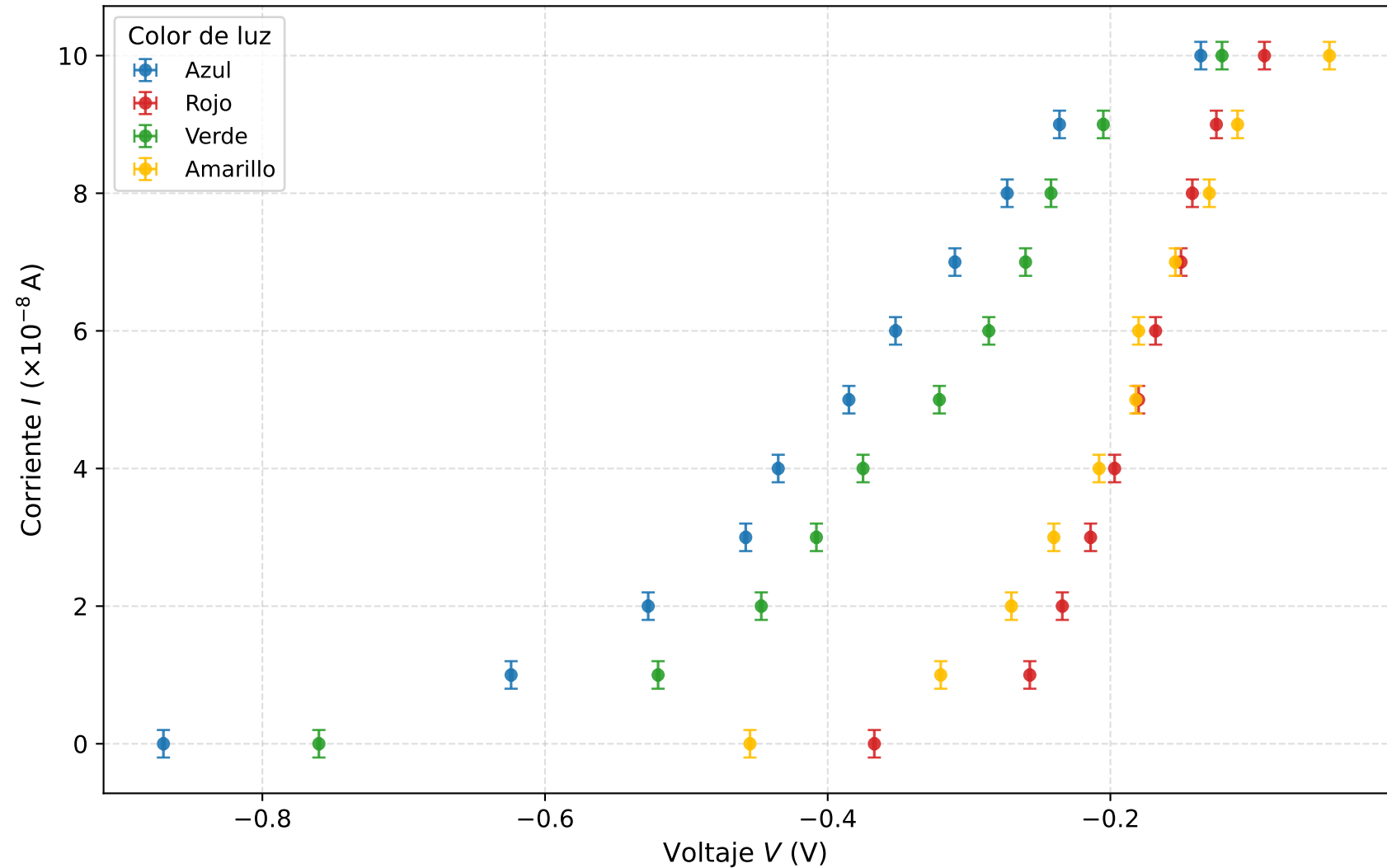
Efecto fotoeléctrico: intensidad vs voltaje
