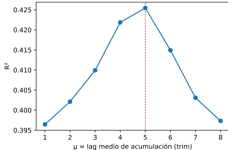
Media del lag SÍ se identifica (óptimo \mu \approx 5q \approx 1 año)
