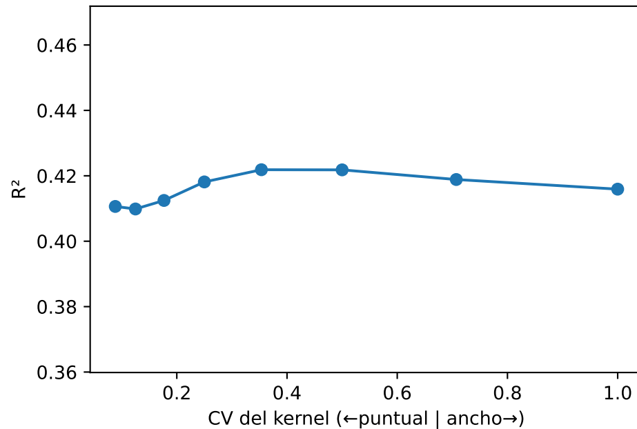
Ancho NO se identifica ( R^2 plano, rango=0.012)
