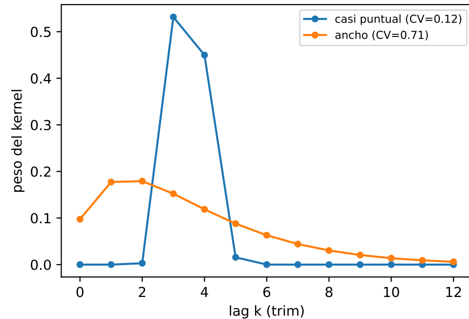
Dos kernels que ajustan IGUAL (indistinguibles con esta data)
