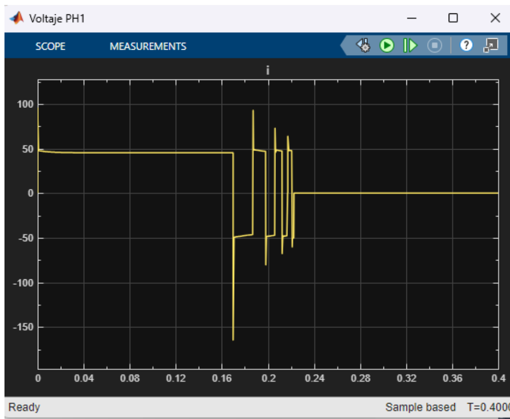
Figura 19: Voltaje de salida del puente H.
