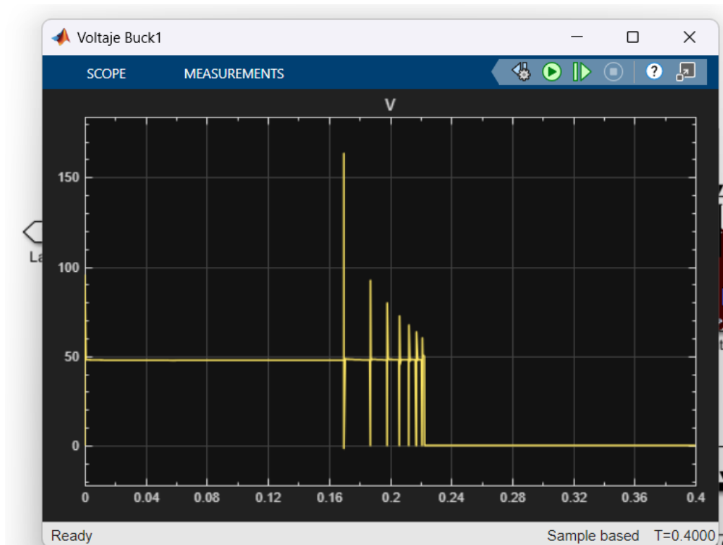
Figura 17: Voltaje de salida del convertidor Buck.
