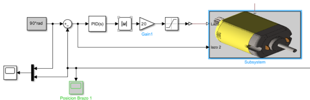
Figura 11: Implementación del lazo cerrado con PID.
