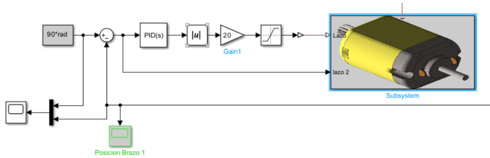
Figura 1: Esquema de control en lazo cerrado.
