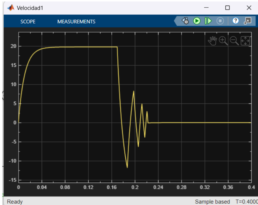
Figura 14: Velocidad angular de la articulación.
