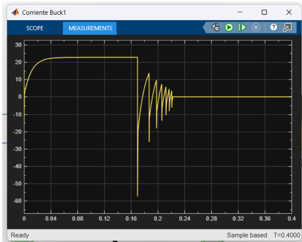
Figura 18: Corriente del convertidor Buck.
