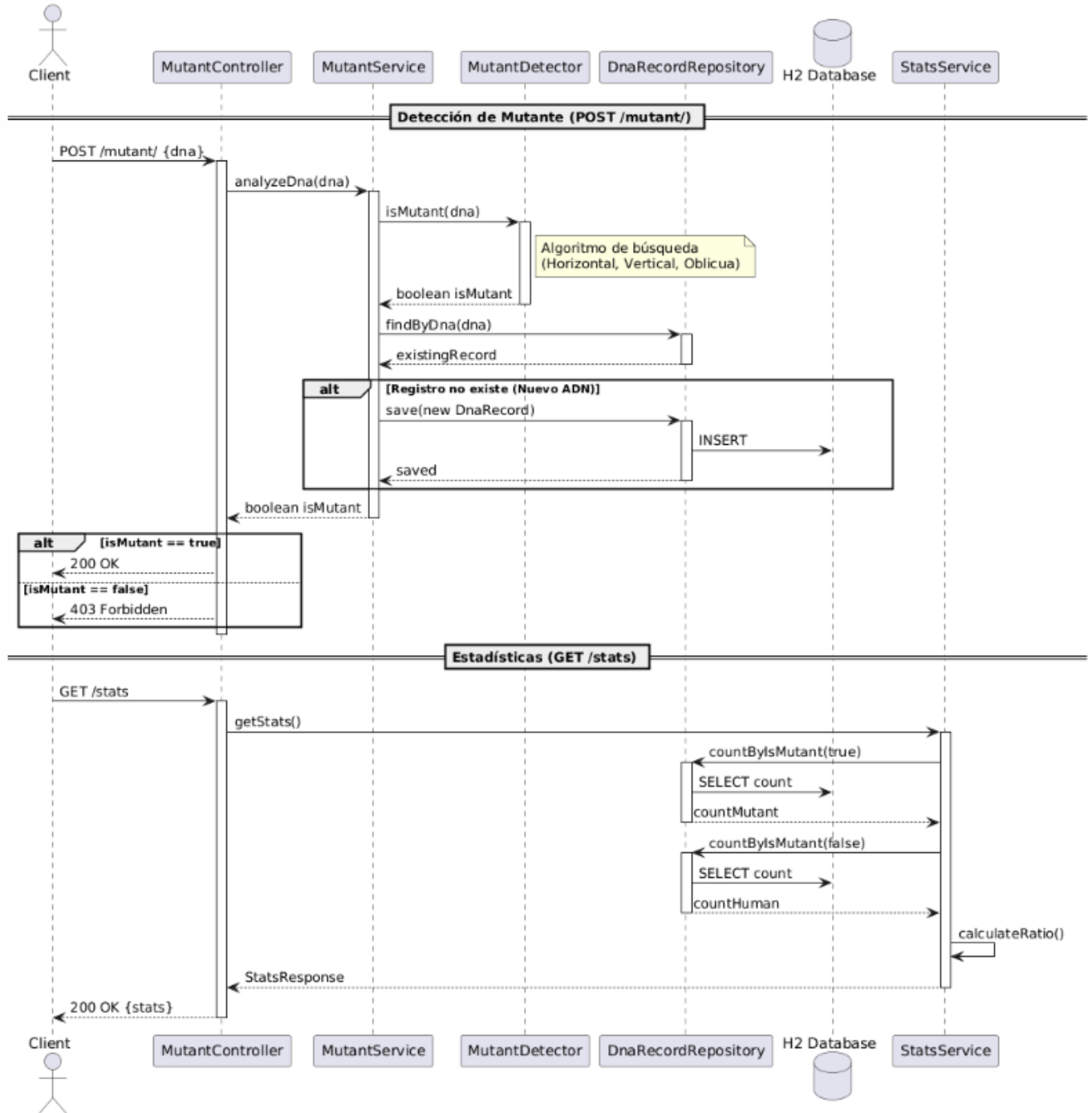
Diagrama de Secuencia - Mutant Detector
