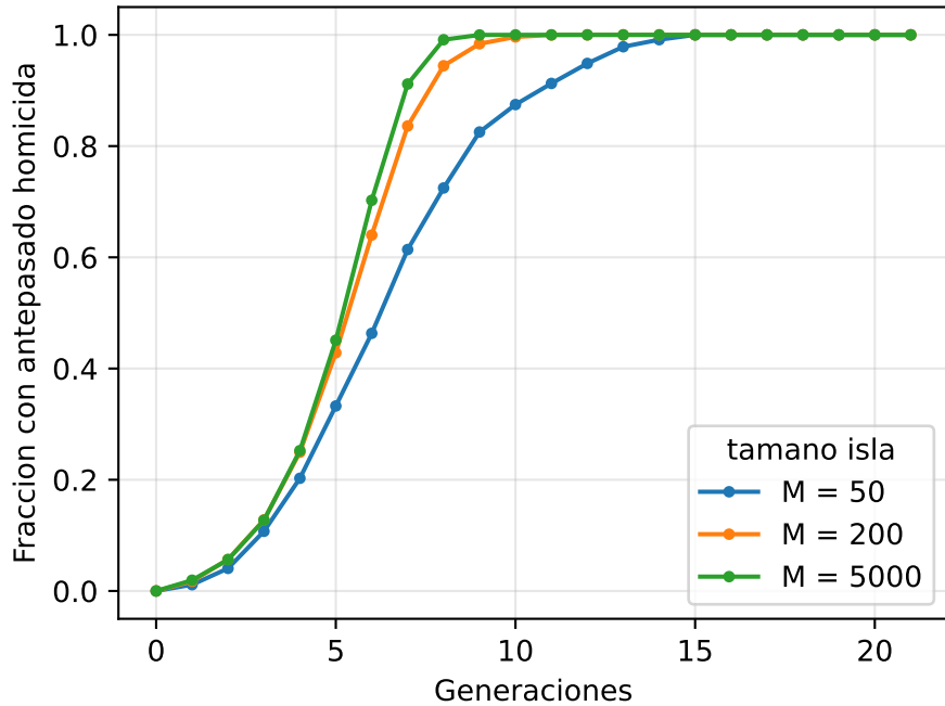
Efecto fundador ( p = 0.01 )
